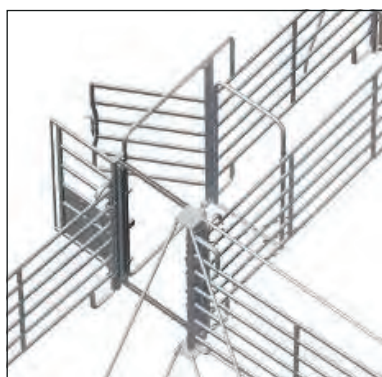
Aufbaubeispiel
