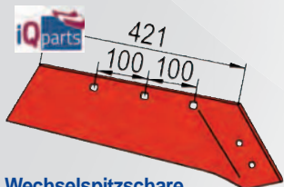
Wechselspitzschare zu V&N WSM43 re. PK801301 Best. Nr. 52447
