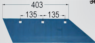
Scharblatt SB-56 re. 3352034 zu Lemken Best. Nr. 52346
