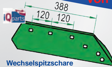
Wechselspitzschare re. 073056 zu Kverneland Best. Nr. 52276
