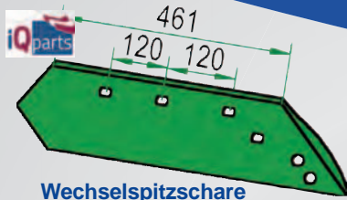
Wechselspitzschare re. 073080 zu Kverneland Best. Nr. 52278
