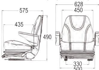
Nr. Bezeichnung 53018 Stapler und Baumaschinensitz mit Bezug Kunstleder schwarz Katalogseite 7
