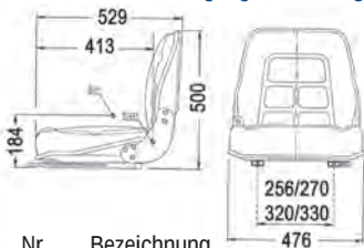
Nr. Bezeichnung 38026 Stapler und Baumaschinensitz mit Bezug Kunstleder schwarz und Totmannschalter eingebaut Katalogseite 6
