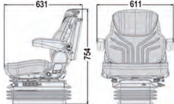
Nr. Bezeichnung G5304 Grammer Maximo Comfort Plus Katalogseite 4
